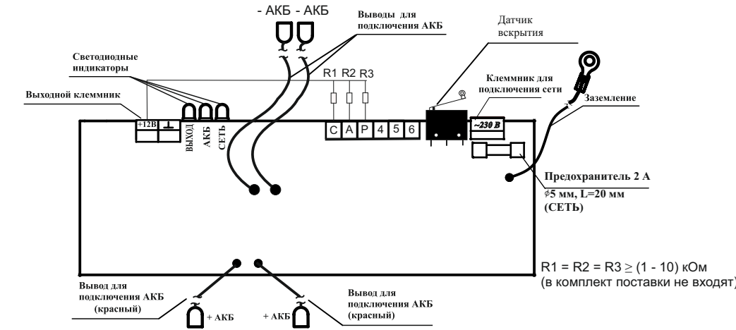
Рисунок 1 - Плата источника
