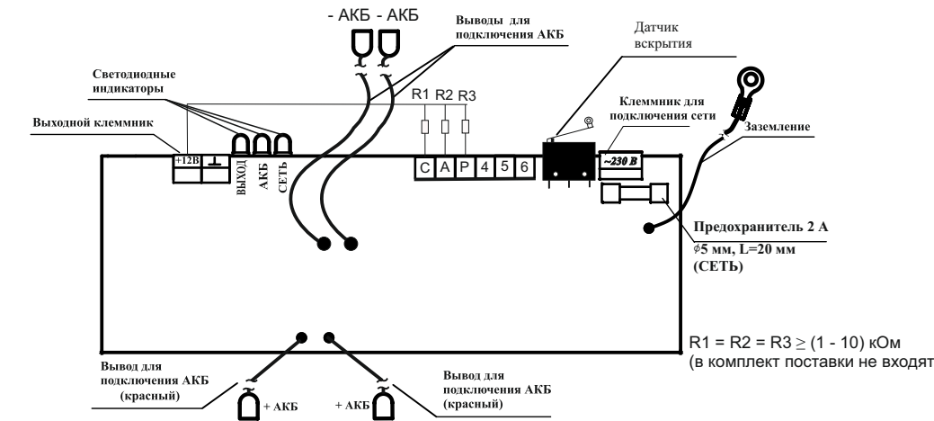
Рисунок 1 - Плата источника
